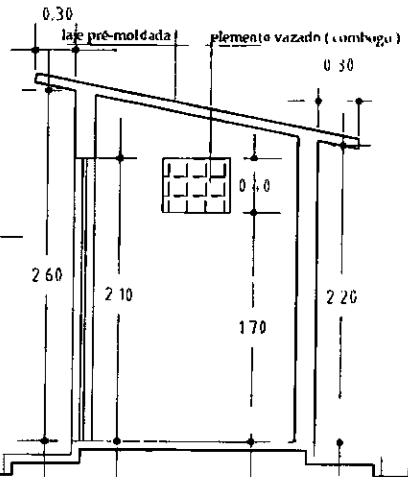
CORTE AB
